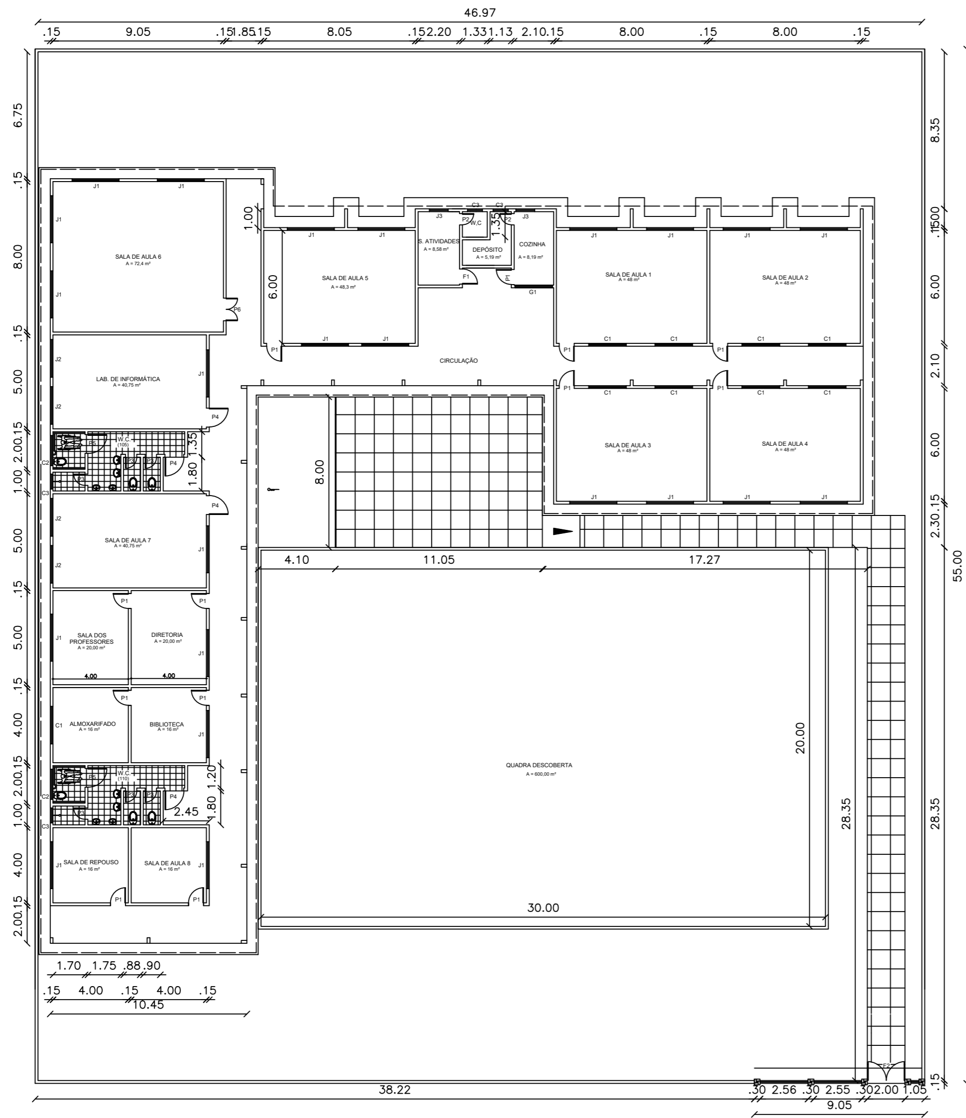
1 PLANTA BAIXA ESCALA 1:200
