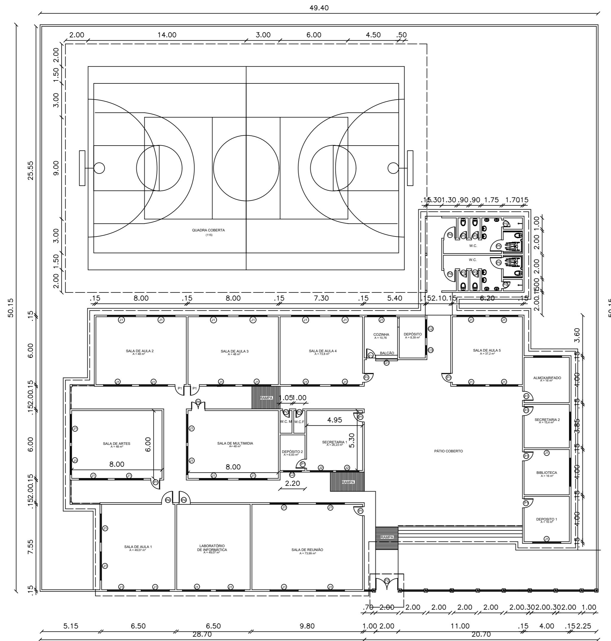
1 PLANTA BAIXA ESCALA 1:200
